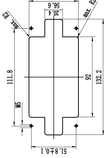
安装开孔图 Panel cut out
